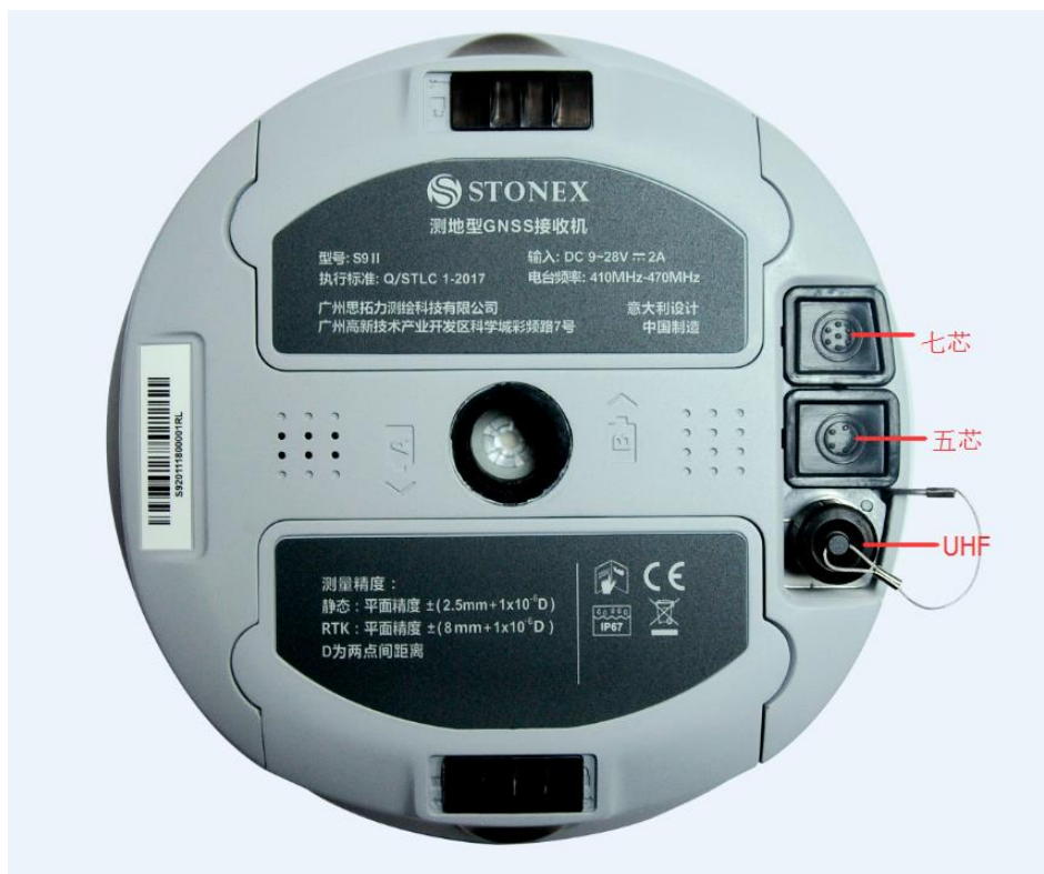
图 3 主机底部
